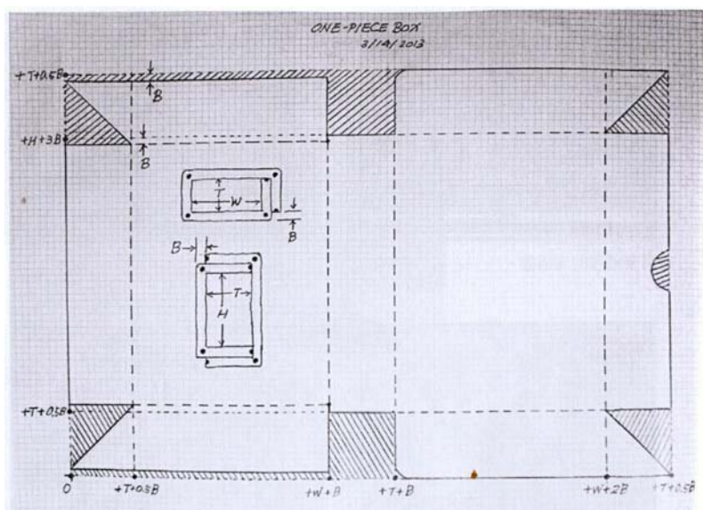
SOP 怎麼寫？還真有學問在。這麼簡單的紙盒圖樣，還有爭論：蓋子畫在左邊還是畫在右邊？各段的長度該個別標示還是累積標示？
